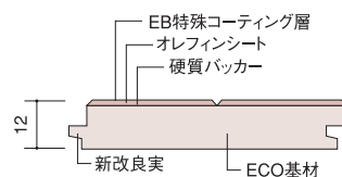
断面図
